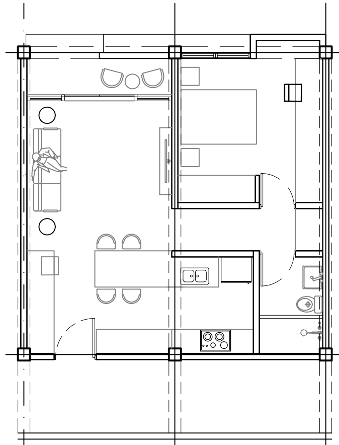
APARTAMENTO DE 1 HABITACIÓN TAMAÑO: 625 PC
