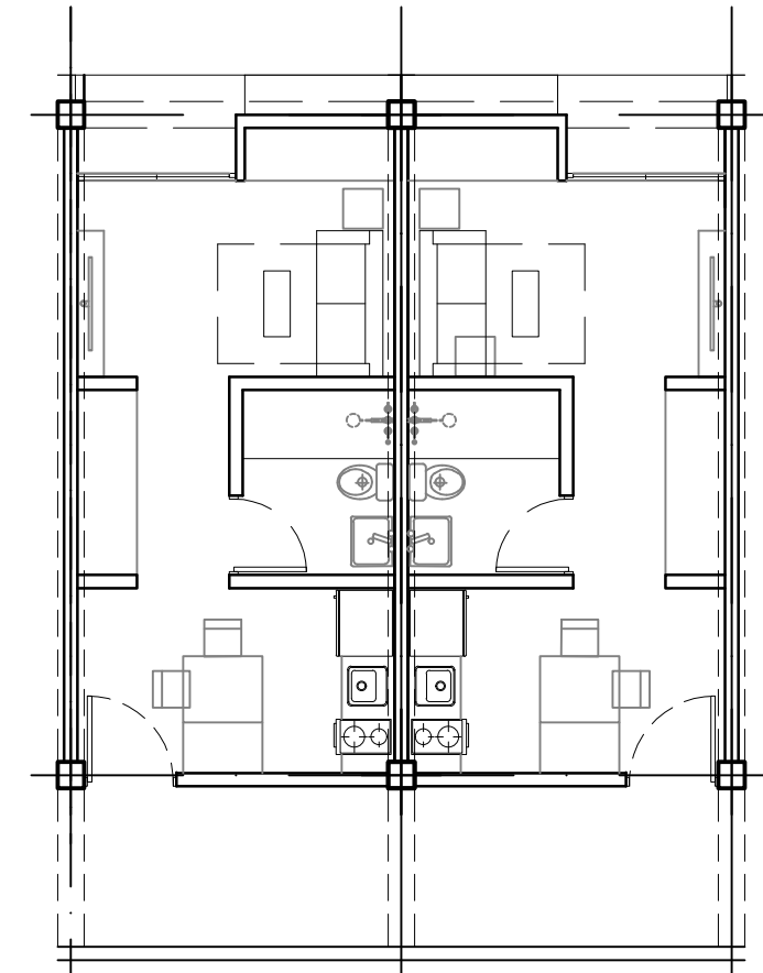
APARTAMENTO DE 1 HABITACIÓN TAMAÑO: 300 PC
